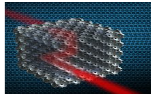
Оптические вычисления
